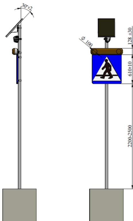
Rys. 3. Rysunek montażowy znaku D-6 z aktywnym panelem
