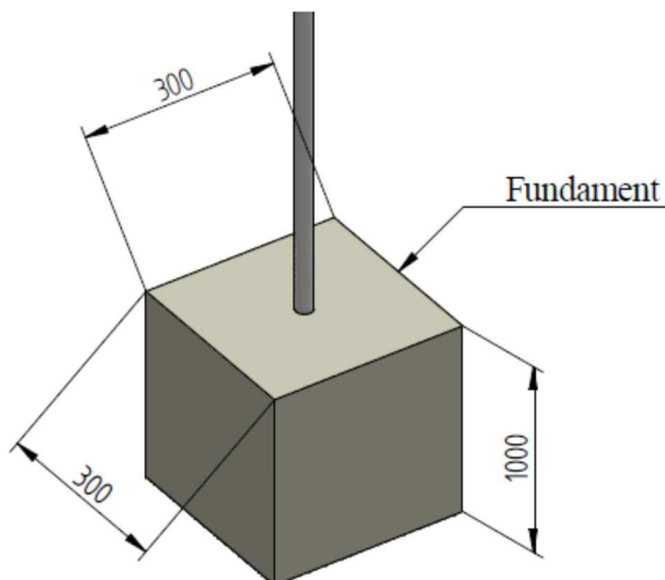
Rys. 4. Wymiary fundamentu
